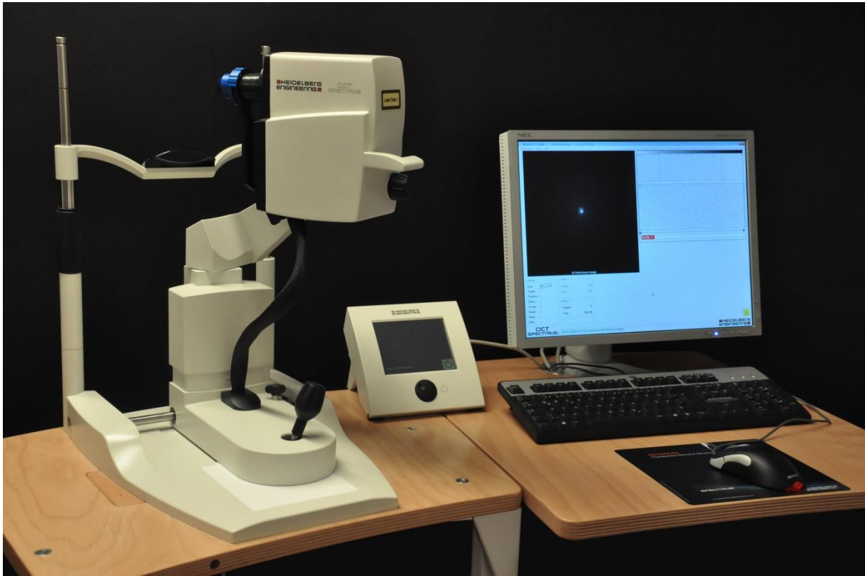
Abbildung 4: SPECTRALIS® HRA+OCT
