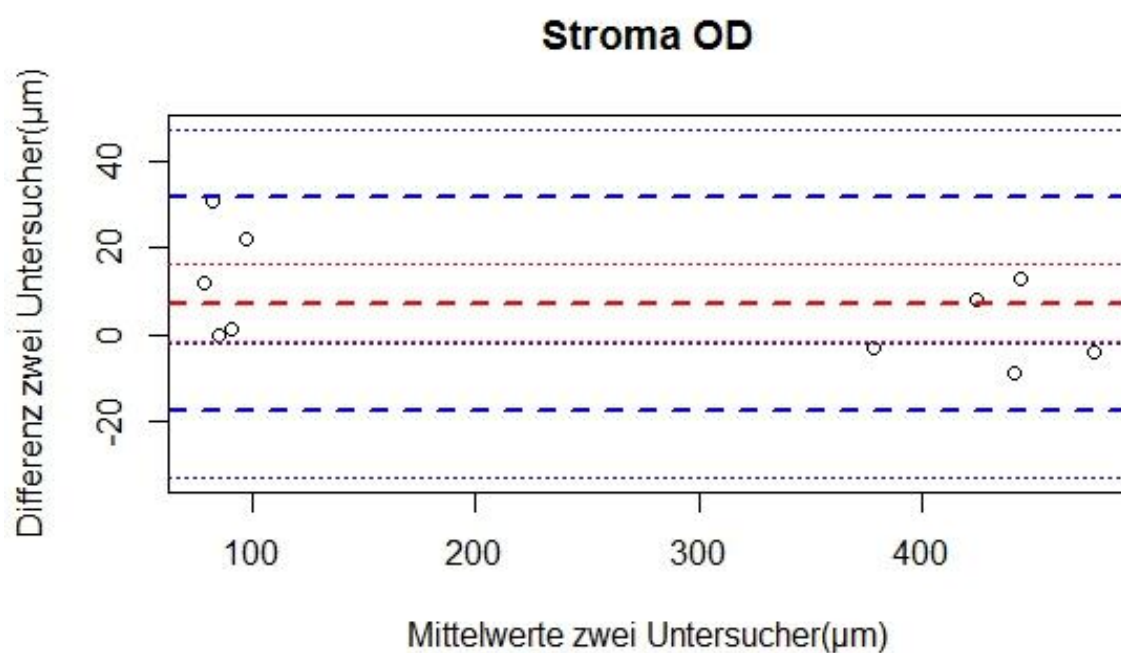
Abbildung 72: Benutzerabhängige Reproduzierbarkeit Stroma OD
