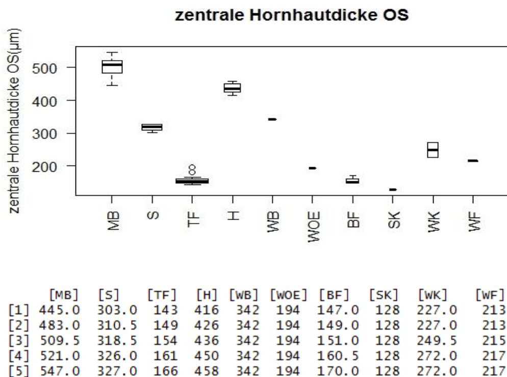
Abbildung 29: Zentrale Gesamtdicke der Hornhaut OS der verschiedenen Arten in μm
